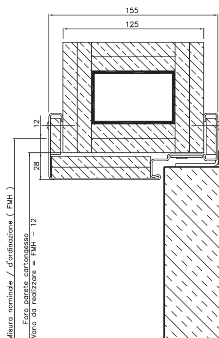
Sezione verticale
